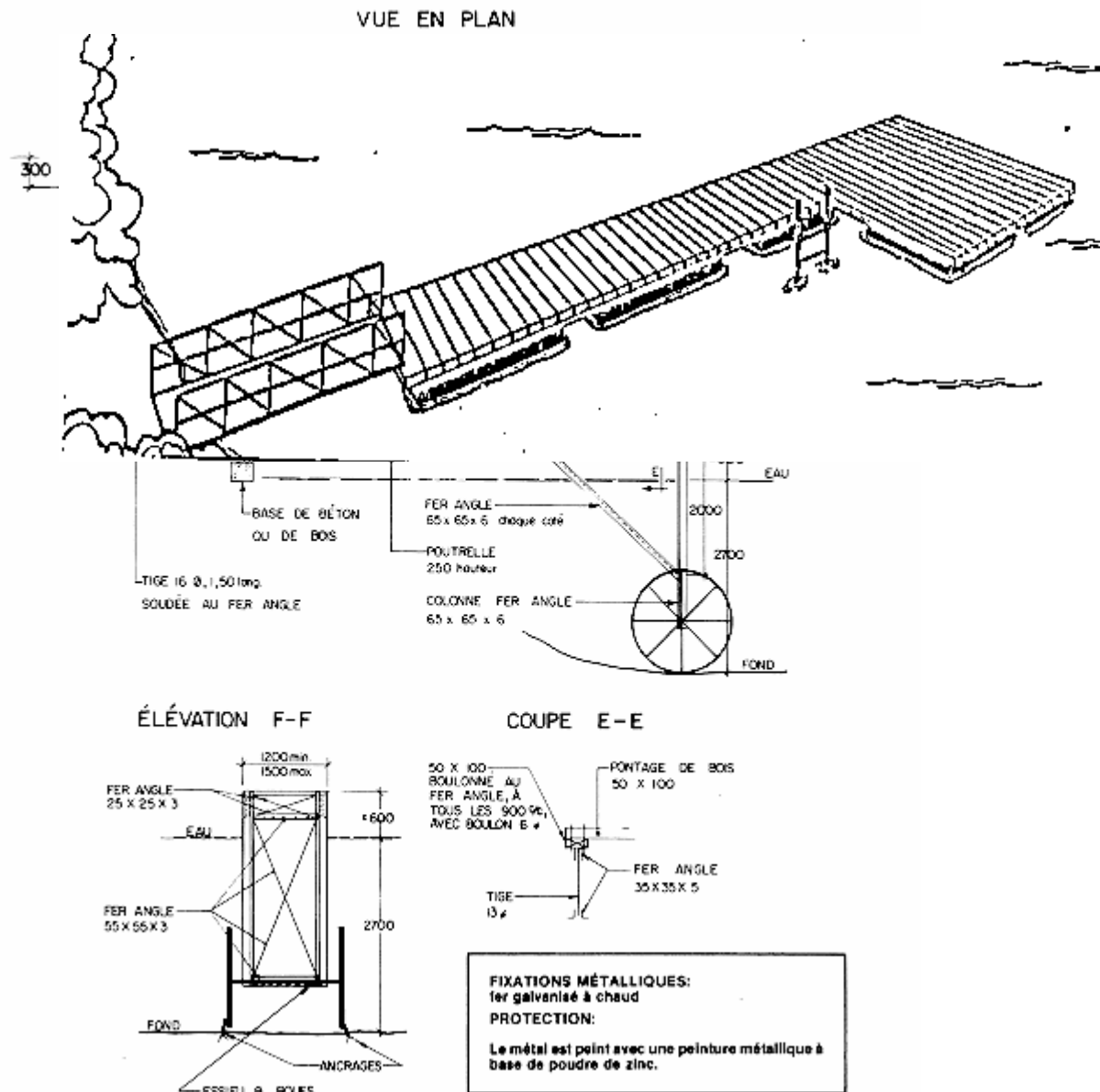
Figure 9.9.4b : Embarcadère amovible roulant, construit sur place
